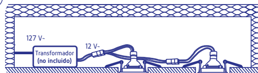
Diagrama para instalar una lámpara a 12 V - lamp Diagram for installing a 12 V - lamp
