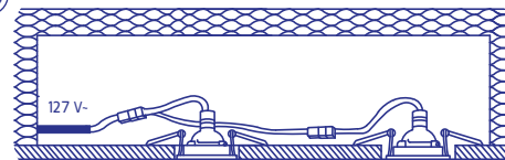
Diagrama para instalar una lámpara a 127 V- Diagram to install a lamp at 127 V -
